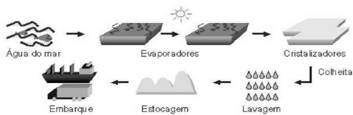
Figura 3: Processo de produção do sal marinho
